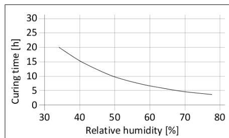
Διάγραμμα 1: Χρόνος ωρίμανσης για φιλμ πάχους 500 μm
